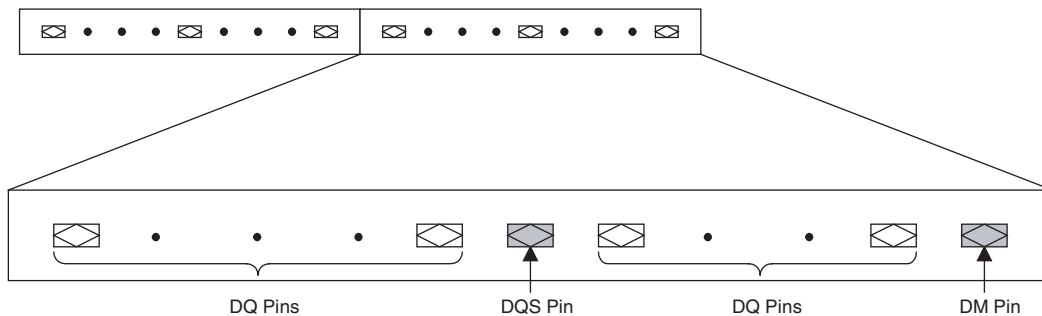
Figure 9-3. Cyclone III DQ and DQS Pins Notes (1), (2), (3), (4)
